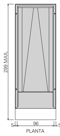
NICHO NVA1-E PESO APROX. : 1430 Kgs.
