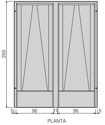
NICHO NVA2 PESO APROX. : 2740 Kgs.
