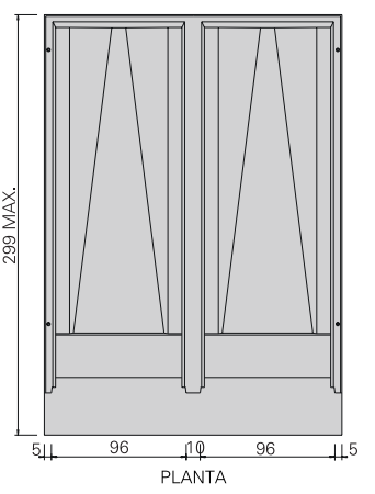
NICHO NVA2-E PESO APROX. : 2860 Kgs.
