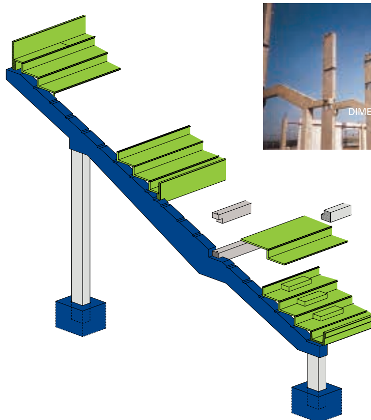
POUTRE LIMON SPÉCIALE AVEC PASSAGE INTERMÉDIAIRE ET AVEC PORTE-À-FAX SUPÉRIEUR
