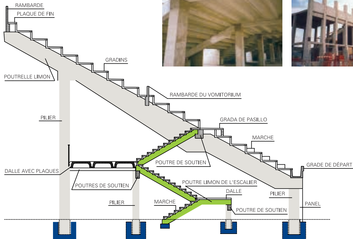
DÉTAIL DES GRADINS AVEC STRUCTURE PRÉFABRIQUÉE.
