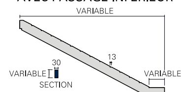
POUTRE LIMON STANDARD AVEC PASSAGE INFÉRIEUR
