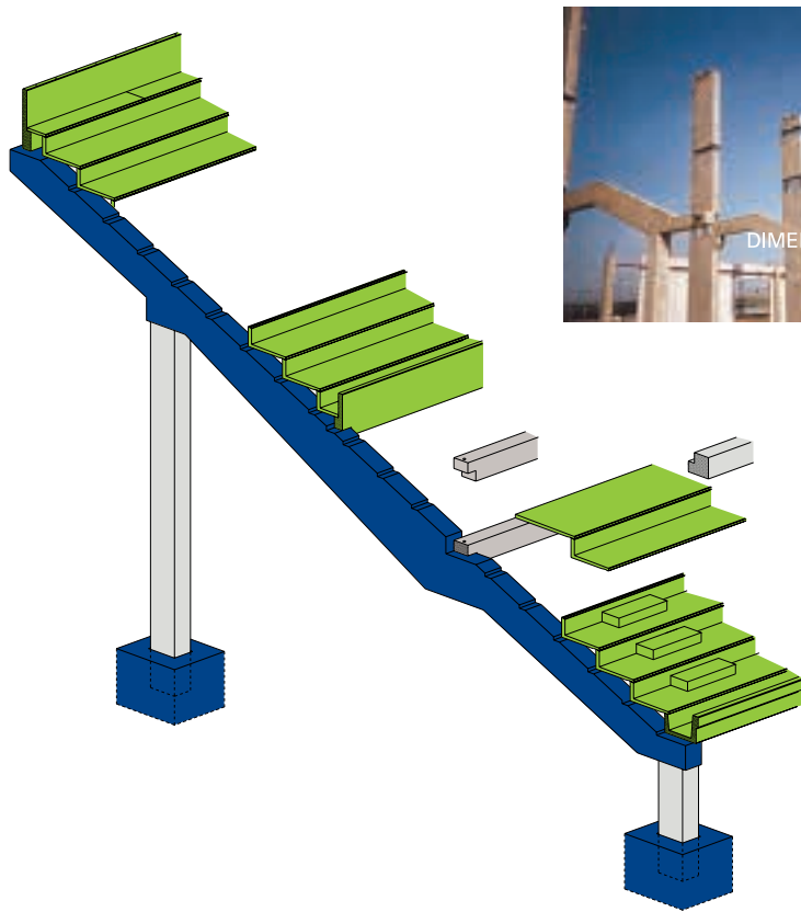
POUTRE LIMON SPÉCIALE AVEC PASSAGE INTERMÉDIAIRE ET AVEC PORTE-À-FAUX SUPÉRIEUR
