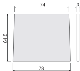
PESO APROX. : 33 Kgs. TAPA INTERIOR DE NICHOS NV1 Y NV2
