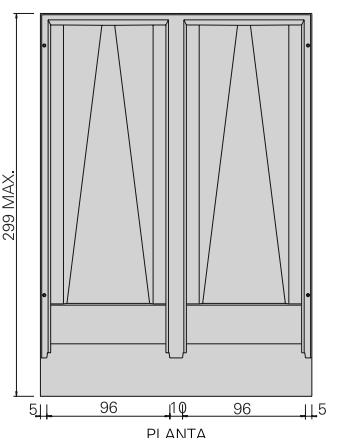
NICHO NVA2-E PESO APROX. : 2860 Kgs.
