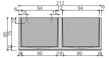
ALZADO
