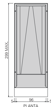
NICHO NVA1-E PESO APROX. : 1430 Kgs.
