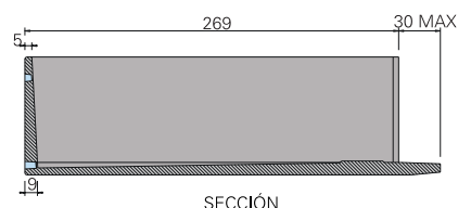
SECCIÓN
