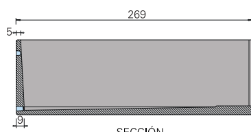
SECCIÓN
