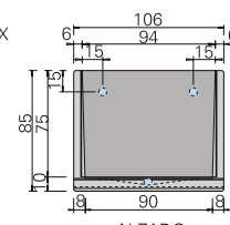
ALZADO
