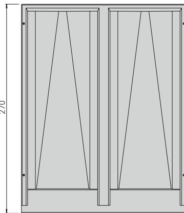
ALZADO
