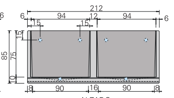
ALZADO
